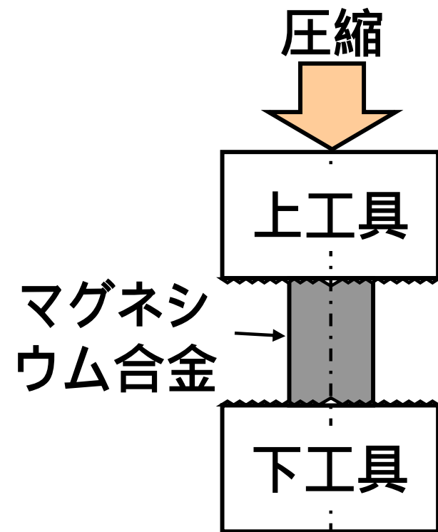
(a) 初期状態 (b) 割れ (c) マッシュルームのような不安定な変形 (d) 樽型の変形
